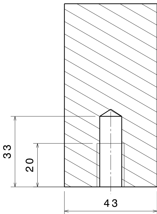
Coupe A-A
